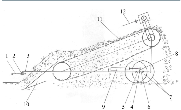
Նկ. 1. Կարտոֆիլահան մեքենայի տեխնոլոգիական սխեման. 1 - կցման սարք, 2, 4 - հողակապեր, 3 - շրջանակ, 5 - երկծունկ սռնի, 6 - ծունկ, 7 - հենարանային անիվներ, 8 - կալունակ, 9 - հիդրոզլան, 10 - խոփ, 11 - էլևատոր, 12 - շարժաբեր մեխանիզմ:
