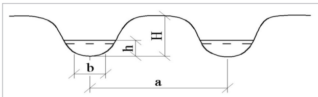
Նկ. 2. Ակոսի սխեման:
