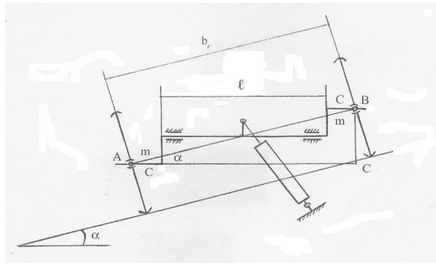
Նկ. 2. Ծնկի երկարության որոշման սխեման:
