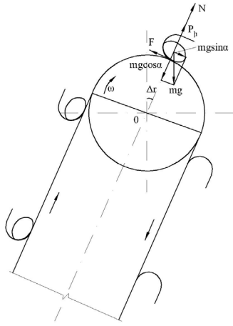
Նկ. 3. Պալարների անկման \alpha_{\min} և \alpha_{\max} անկյունների համապատասխան հետագծերի սխեման:
