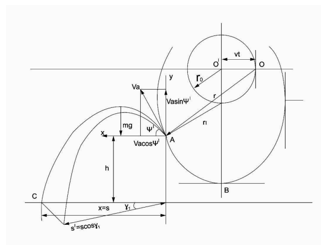
Նկ. 2. Հողային տաշեղի թռիչքի հետագոտության հաշվարկային սխեման (կազմվել է հեղինակների կողմից):
