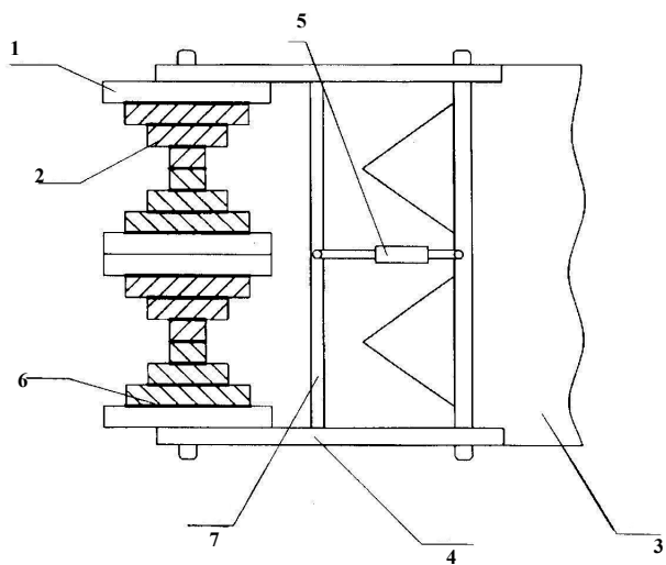
Նկ. 1. Կոշտամանրիչ-փոխակրիչի սկզբունքային սխեման. 1 - ռոտոր, 2 - դանակ, 3 - կարտոֆիլահան մեքենա, 4 - հողակապով լծակ, 5 - կարգավորիչ հարմարանք, 6 - օղագոտի, 7 - հորիզոնական ձող (կազմվել է հեղինակների կողմից):
